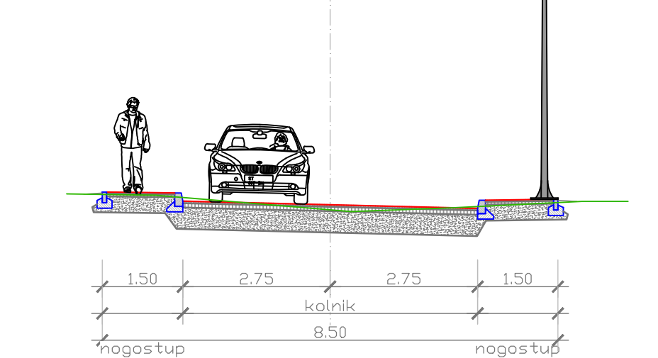
KARAKTERISTIČNI POPREČNI PRESJECI PLANIRANIH ULICA MJ 1:100 PRESJEK A
