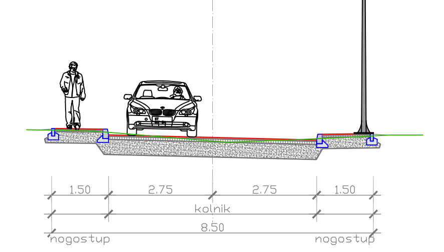
PRIJEDLOG KARAKTERISTIČNIH POPREČNIH PRESJEKA PLANIRANIH ULICA MJ 1:100 PRESJEK A
